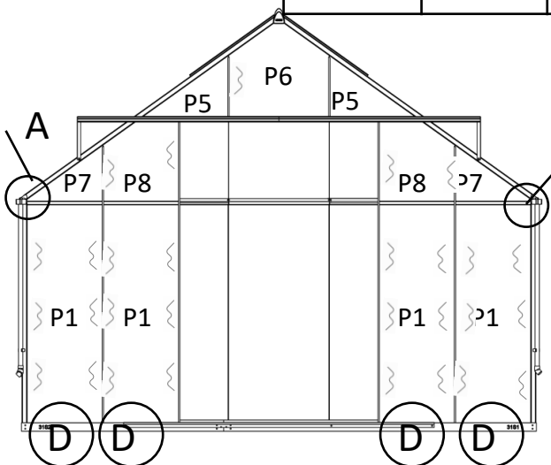
Čelní pohled / Čelný pohľad / Widok od przodu / Vorderansicht
