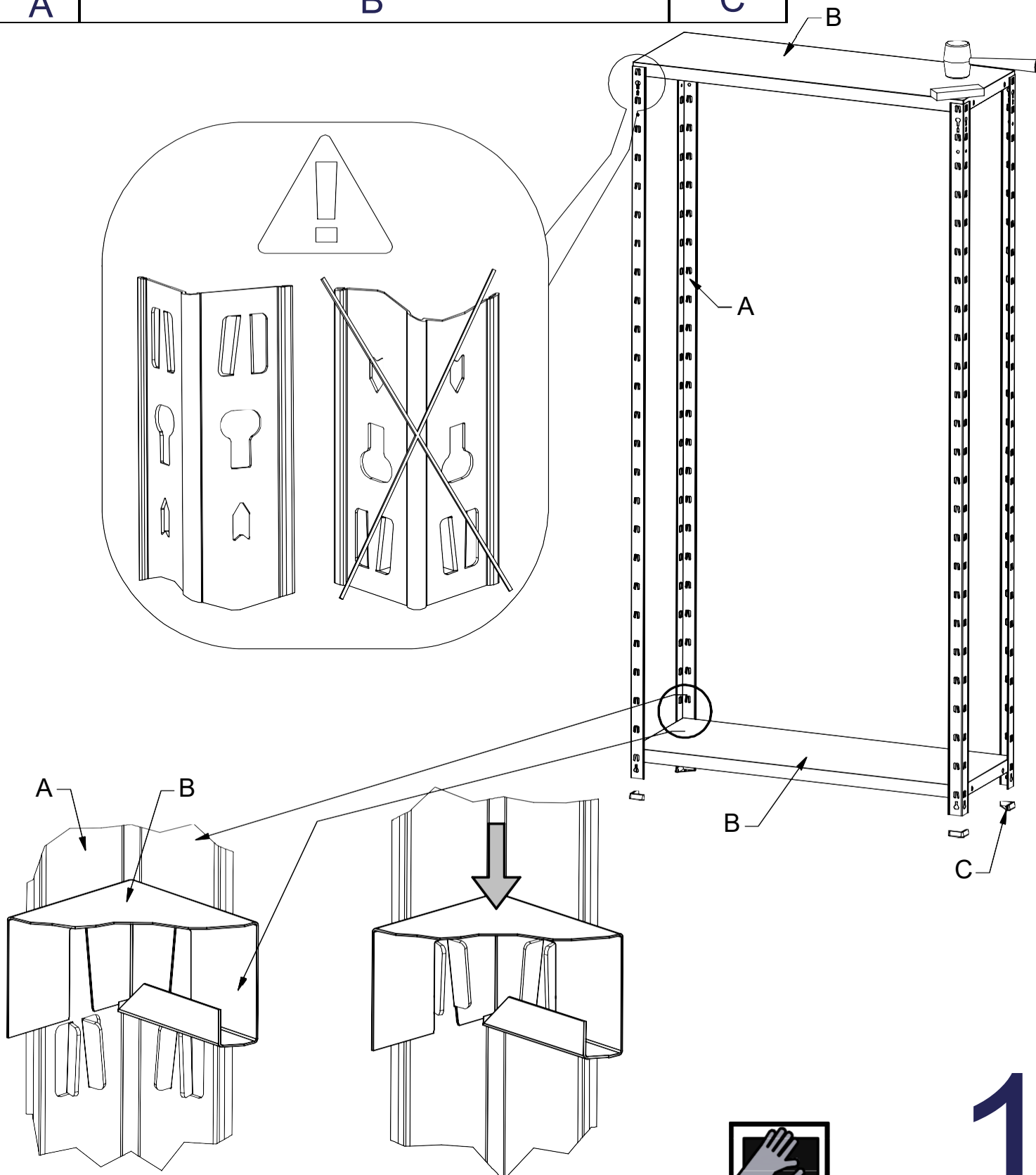
DETAL MOCOWANIA PÓŁKI W REGALE
