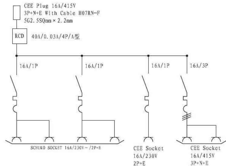
Schemat blokowy połączenia elektrycznego
