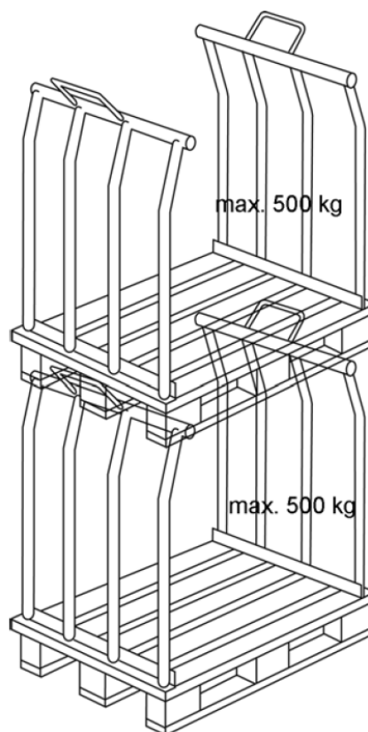
Rys. 8 udźwig przy układaniu w stos maks. po 500 kg
